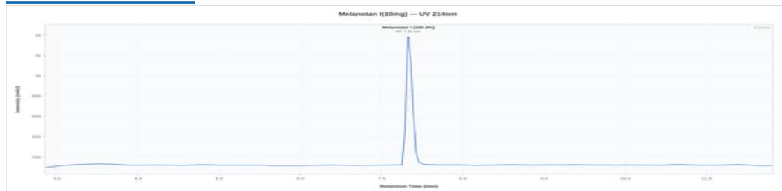
Melanotan I 10mg - MT01-02: UV Chromatogram
